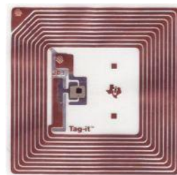
Gambar 1. RFID Tag
