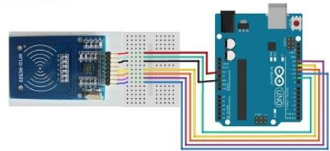
Gambar 9. Instalasi Arduino Uno dengan RFID Tag
