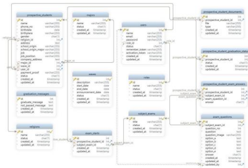
Gambar 4.4 Rancangan Database
